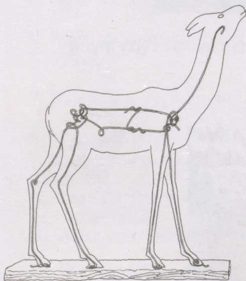
Каркастын схемасы.
