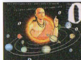
Астрономдор Айдын фазаларын жана Жер өз огунда айланарын аныкташкан.
