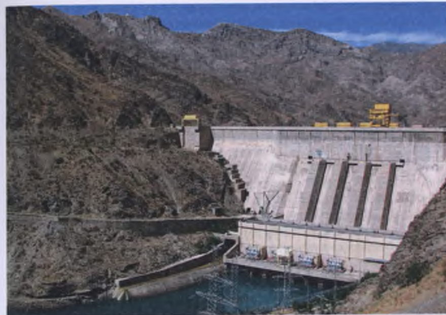
Курпсайская ГЭС
