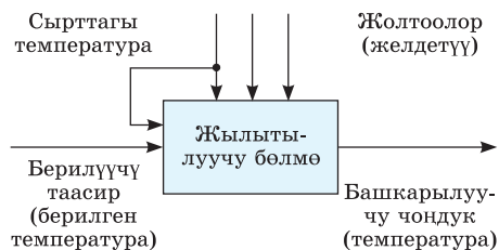
46-сүрөт. 45-сүрөттөгү көзөмөлдөөчү системанын функциялык схемасы.
