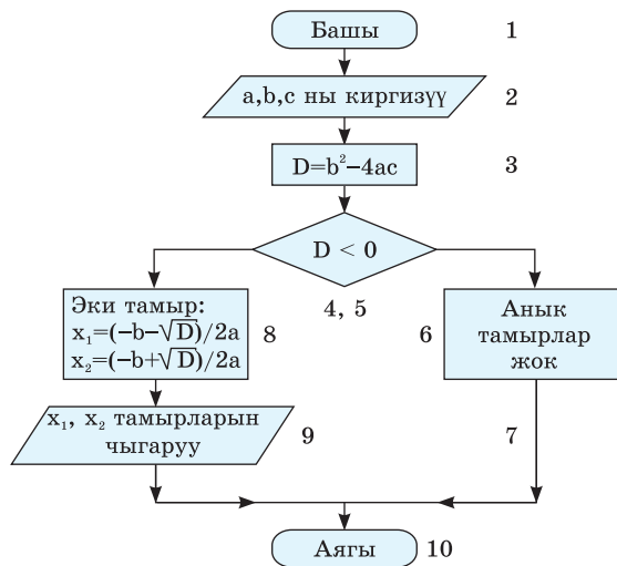
56-сүрөт. Алгоритмдин блок-схемасы.
