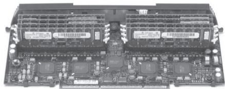
89-сүрөт. Системалык плата.
