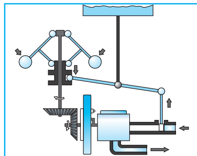
35-сүрөт. Валдын айлануу жыштыгын автоматтык жөндөгүч.
