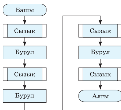
62-сүрөт. «Алкак» алгоритминин блок-схемасы.
