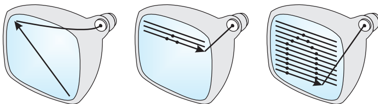
129-сүрөт. Электрон-нур түтүгүндө растрдык сүрөттөлүштү алуу.
