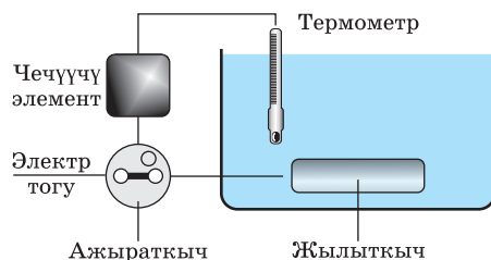
44-сүрөт. Суунун туруктуу температурасын кармап туруучу түзүлүш.
