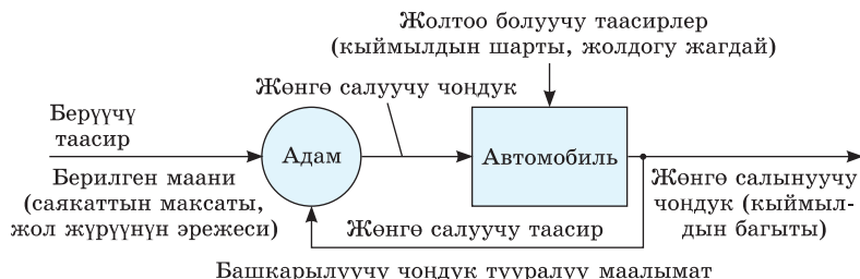
49-сүрөт. Автомобилди башкаруу – жөнгө салуунун туюк контуру.
