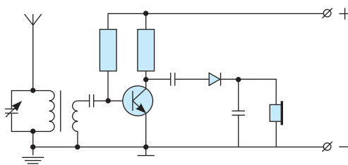
53-сүрөт. Жөнөкөй радиокабылдагычтын принципалдык электр схемасы.
