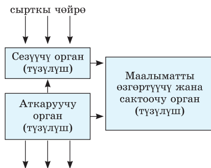
38-сүрөт. Өзү башкарылуучу системанын жөнөкөйлөтүлгөн схемасы.
