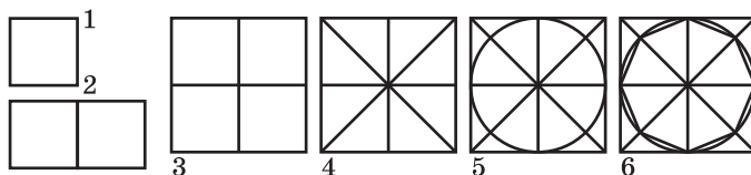
119-сүрөт. Туура сегиз бурчтукту түзүү алгоритми.
