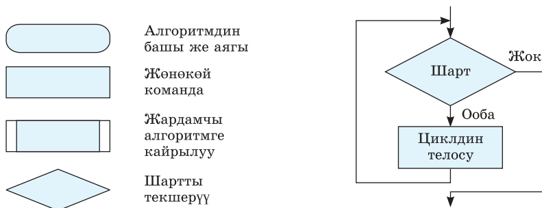
63-сүрөт. Блок-схеманын элементтери жана циклдин структурасы.
