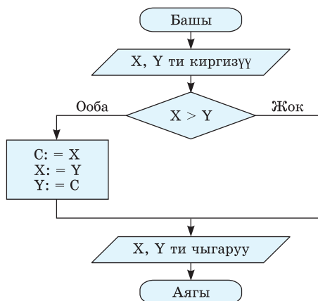
73-сүрөт. Эки чоңдукту иреттөөнүн алгоритми.
