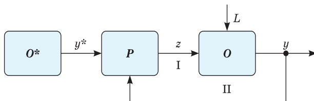
41-сүрөт. Тескери байланыш.
