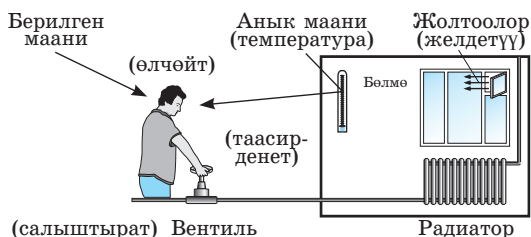
47-сүрөт. Бөлмөдө абанын температурасын жөнгө салуунун принциби.
