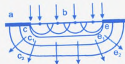
140-сүрөт. Дифракциялык торчонун кандайдыр жылчыгынан (в) өтүү менен (сd) толкун фронтунун кеңейиши (б – чоңойтулуп көрсөтүлгөн учуру).
