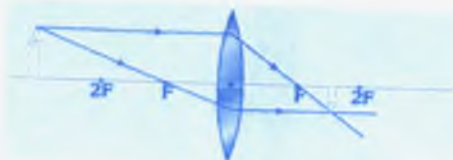
119-сүрөт. Нерсе линзанын кош фокусунан алыс жайгашкан.
