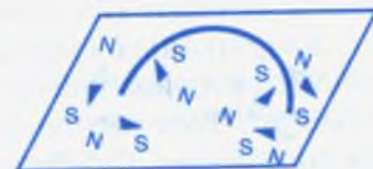
22-сүрөт. Тегерек токтун магниттик күч сызыктарынын багыты.
